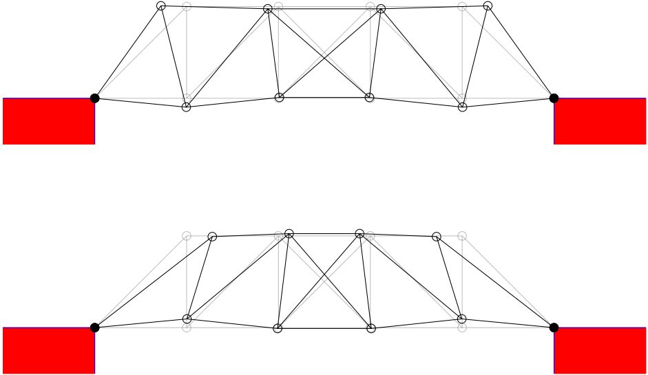
Abb. 22.2: Eine andere Eigenschwingung der Brücke
