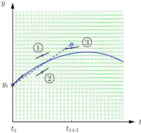
Abb. 76.1: Runge-Kutta-Ansatz
