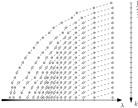
Abb. 30.1: Monotonie-Eigenschaften der Ritzwerte
