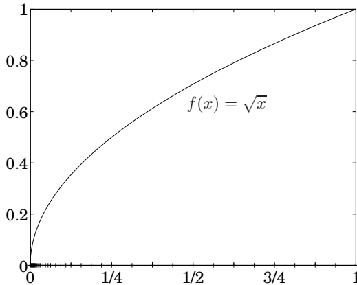
Abb. 42.1: Adaptives Gitter für die Integration von \sqrt{x} .
