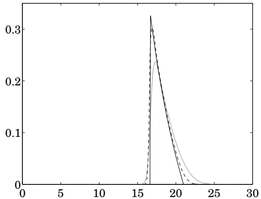
Abb. 110.1: Numerisches Ergebnis des MUSCL-Verfahrens
