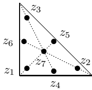
Abb. 93.2: Quadraturformeln mit Exaktheitsgrad q = 3 und q = 5
