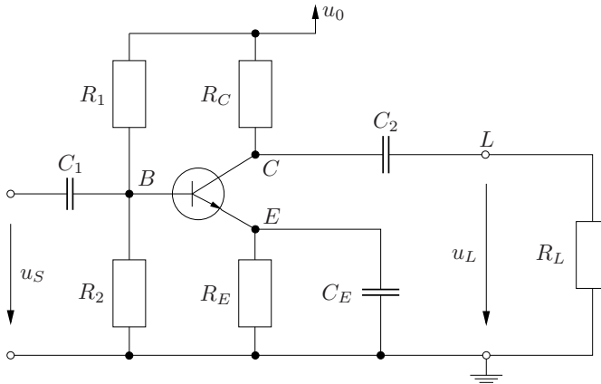
Abb. 64.1: Verstärker-Grundsaltung
