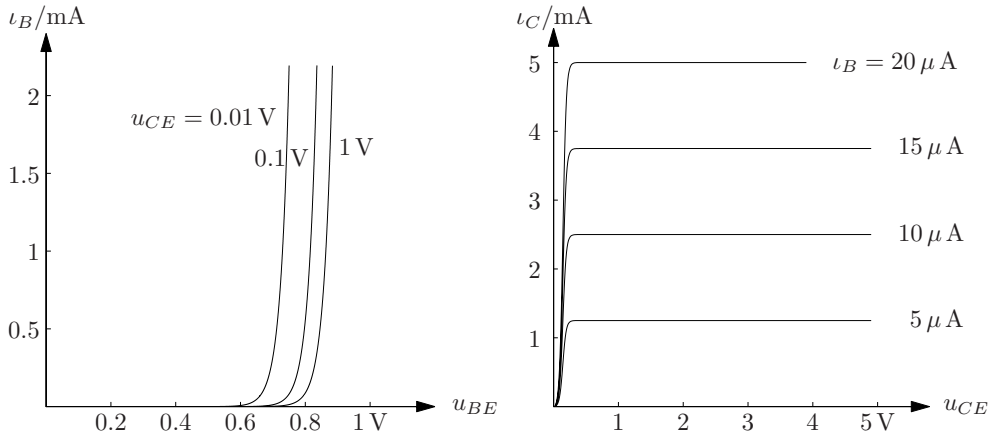
Abb. 64.2: Kennlinien eines Transistors
