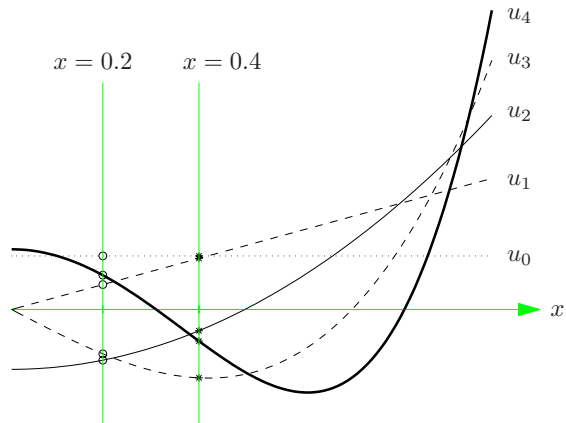
Abb. 35.2: Die Legendre-Polynome und der Satz von Sturm
