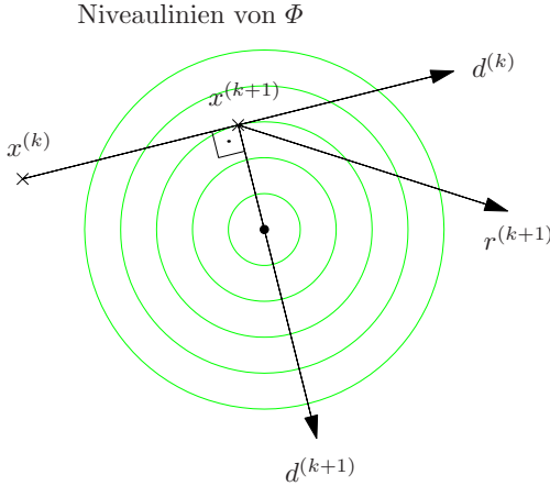
Abb. 9.1: Skizze in der \|\cdot\|_A -Geometrie: d^{(k+1)} ist die optimale Suchrichtung
