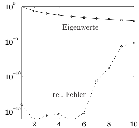
Abb. 30.3: Konvergenzgeschwindigkeit und relative Genauigkeit des Lanczos-Verfahrens
