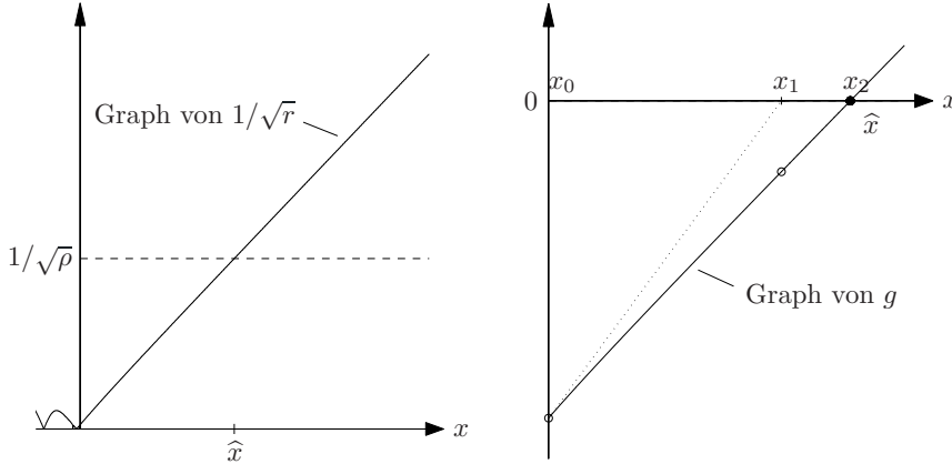
Abb. 18.5: Graph von 1/\sqrt{r} (links) und die Hebden-Iterierten (rechts)
